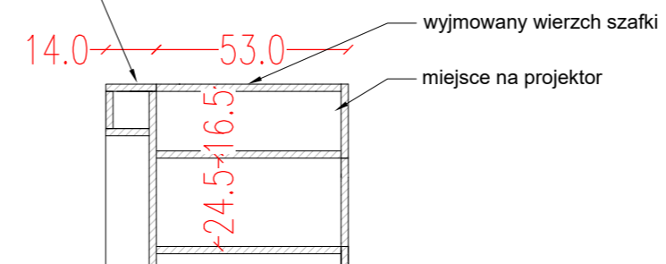
Przekrój A-A
